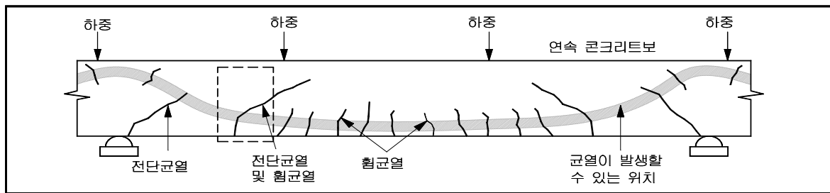
【그림 3.2.5】 콘크리트 거데에 발생하는 균열의 유형과 위치
