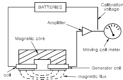
【그림 3.4.3】 전자기유도 방식에 의한 철근탐사장비의 구성
