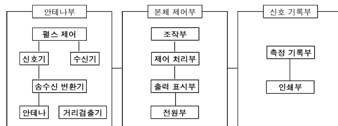
【그림 3.4.4】 전자파 레이더법에 의한 철근탐사장비의 장치 구성도
